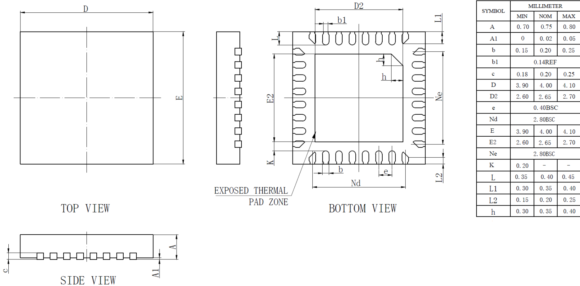
图 3-2 QFB32_4X4 封装尺寸图
